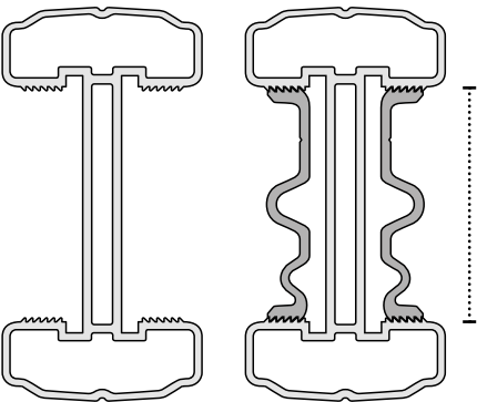
Clip de fixation panneau soudé pour poteau alu 155 - 250 - 450
