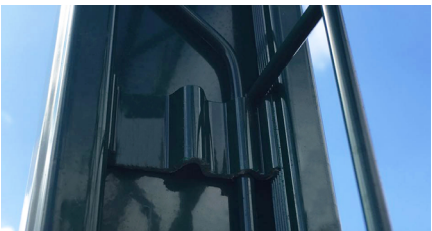
CLIP FIXATION POTEAU/PANNEAU Vis 6x40 + écrou autocassant
